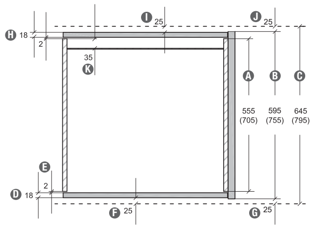
Wangentiefe bei freistehenden Lösungen
