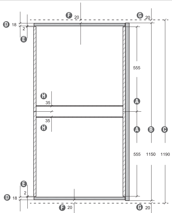
Wangentiefe bei freistehenden Lösungen
