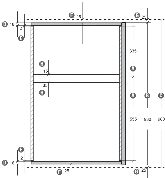
Wangentiefe bei freistehenden Lösungen
