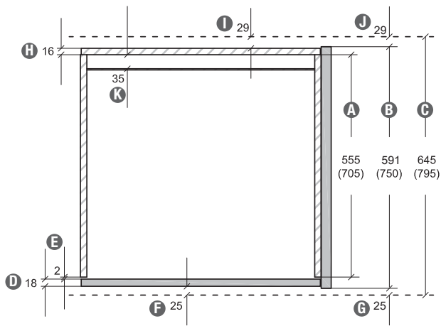
Wangentiefe bei freistehenden Lösungen
