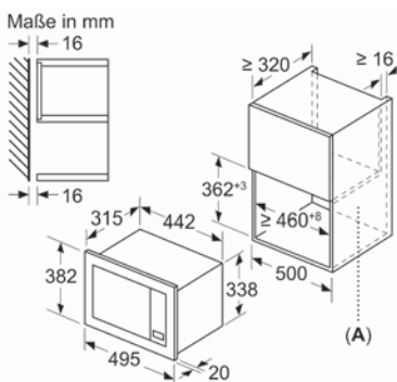
A: Rückwand offen
